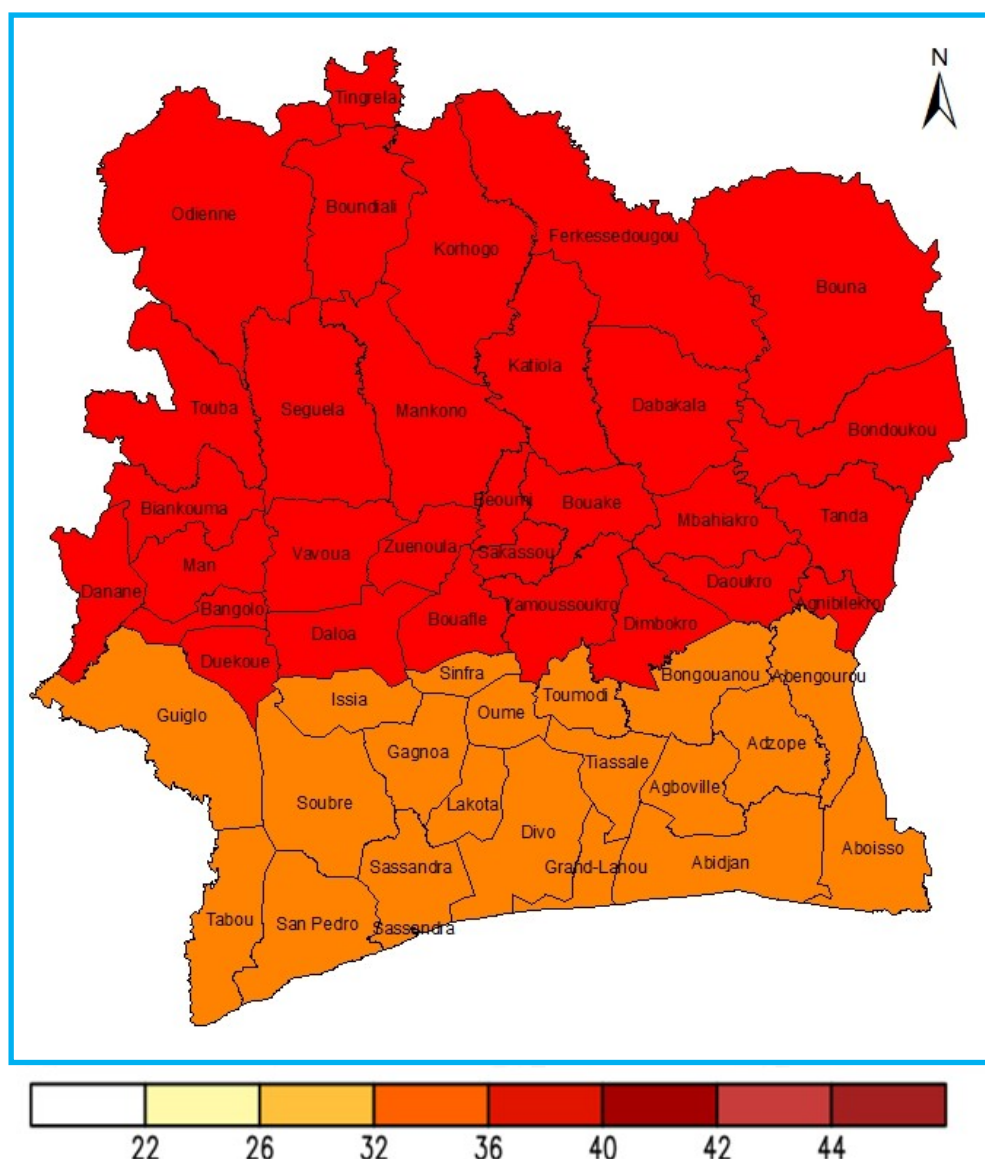
Figure 2: prévision de la température maximale du 02 au 08 Mars 2026
