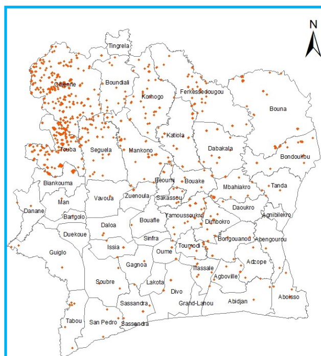
Figure 1 : Foyers de feux actifs détectés du 21 au 28 février 2026 par les satellites MODIS
