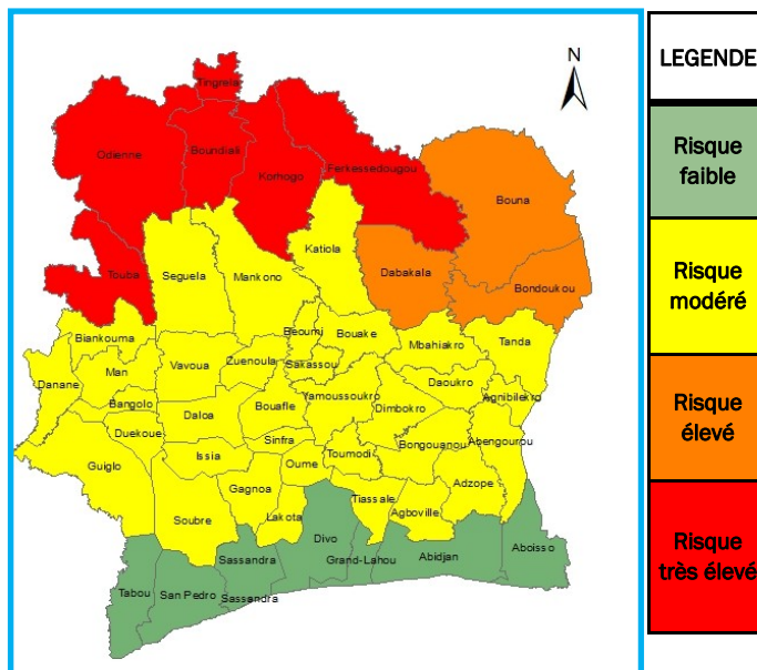
Figure 3: Risque de feux de forêt du 01 au 10 Mars 2026
